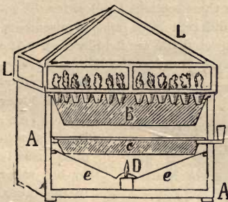
Fig. 34. Propagating-oven.
